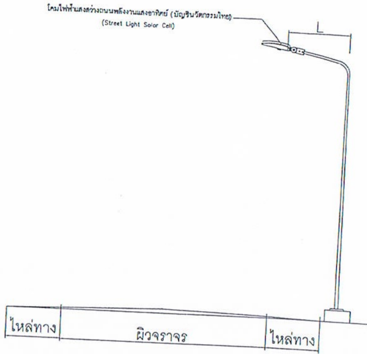
L - ระยะจากเสาไฟถนนถึงขอบผิวจราจร (ศูนย์กลางของดวงโคมอยู่ตรงกับขอบผิวจราจร) รูปแบบการติดตั้งเสาไฟทำแสงสว่างถนนพลังงานแสงอาทิตย์บริเวณ ไหล่ทาง
