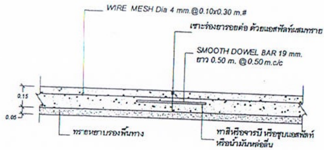
DETAIL. CONSTRUCTION JOINT (รอยต่อเพื่อการก่อสร้าง) SCALE NO.
