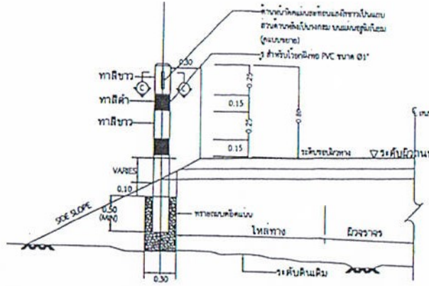
รูปตัด (A)-(A) ไม่แสดงมาตราส่วน
