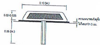
รูปด้านข้างปริมสะท้อนแสง ไม่แสดงหารั้ว
