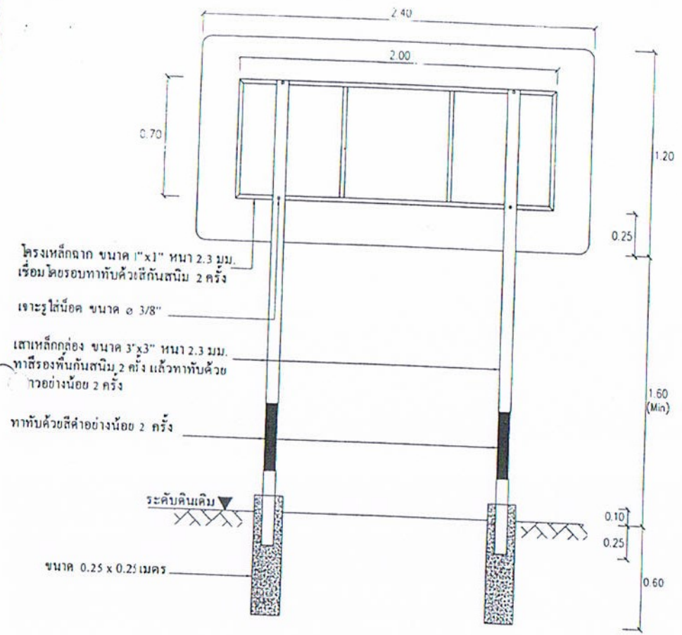
รายละเอียดด้านหลังป้าย
