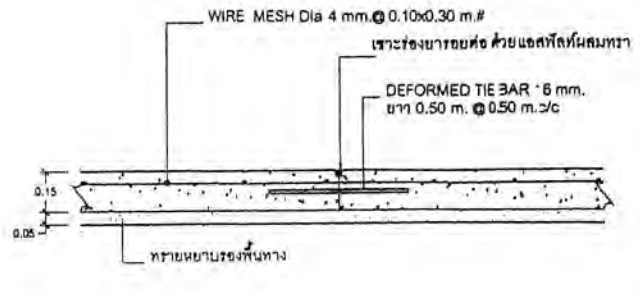
DETAIL 2. LONGITUDINAL JOINT (รอยต่อตามยาว) SCALE NO.
