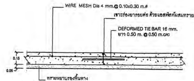
DETAIL 2. LONGITUDINAL JOINT (รอยต่อตามยาว)
