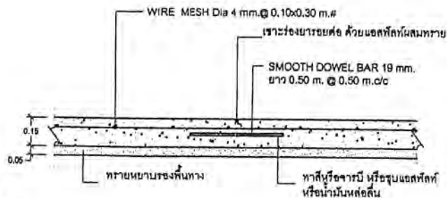
DETAIL. 1. CONSTRUCTION JOINT (รอยต่อเพื่อการหดตัว)
