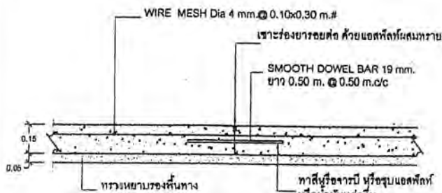
DETAIL. CONSTRUCTION JOINT (รอยต่อเพื่อการก่อสร้าง)
