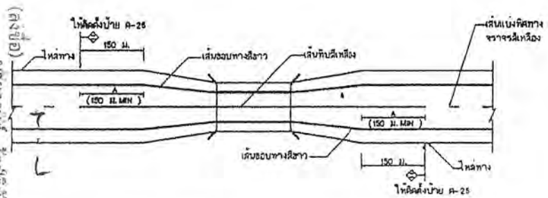
การตีเส้นจราจรกรณีความกว้างสะพานน้อยกว่าความกว้างผิวจราจรบน ไม้ลงคนทางซ้าย
