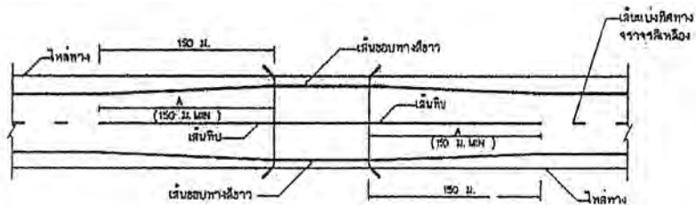
การตีเส้นจราจรกรณีความกว้างสะพานมากกว่าความกว้างผิวจราจรบน ไม้ลงคนทางซ้าย
