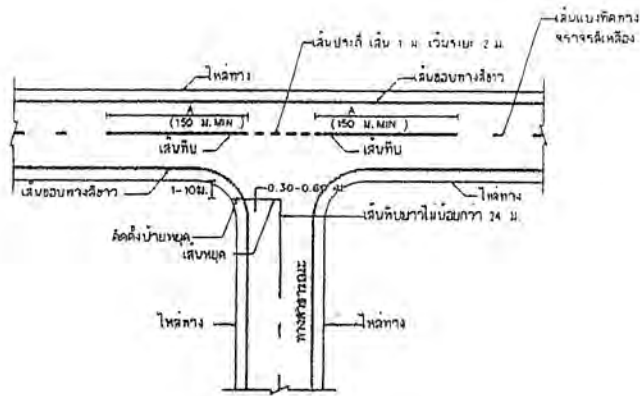
การตีเส้นจราจรทางแยก (ทางมาตรฐาน)
