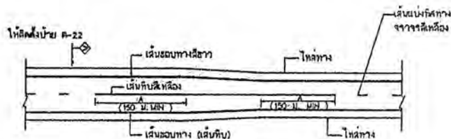
การตีเส้นจราจร กรณีความกว้างของช่องจราจรลดลง ไม้ลงคนทางซ้าย
