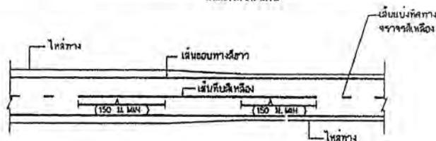
การตีเส้นจราจร กรณีความกว้างของไหล่ทางลดลง ไม้ลงคนทางซ้าย
