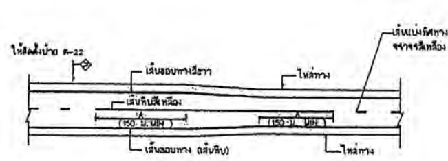
การตีเส้นจราจร กรณีความกว้างของช่องจราจรลดลง ไม่ลดขนาดส่วน
