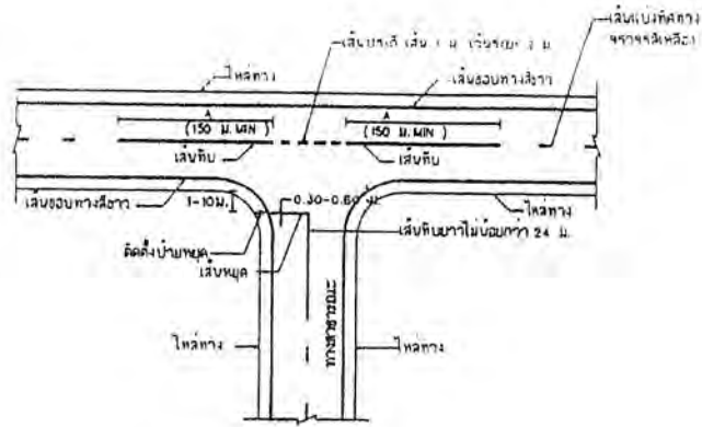
การตีเส้นจราจรทางแยก (ทางสาราณน)
