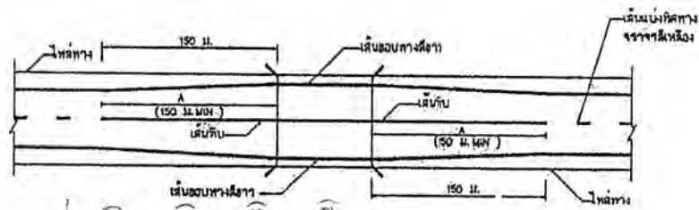
การตีเส้นจราจรกรณีความกว้างสะพานมากกว่าความกว้างผิวจราจรบน ไม่ลดขนาดส่วน
