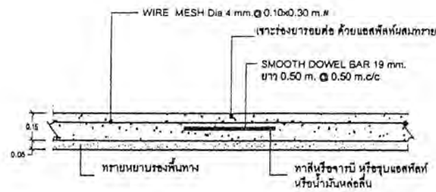
DETAIL. 1. CONSTRUCTION JOINT (รอยต่อเพื่อกำหนดตัว)
