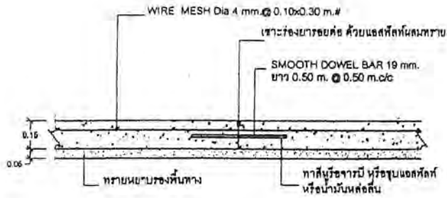
DETAIL. CONSTRUCTION JOINT (รอยต่อเพื่อกำหนดตัว)
