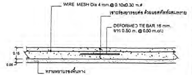
DETAIL 2. LONGITUDINAL JOINT (รอยต่อตามยาว)
