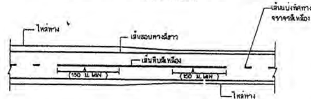
การตีเส้นจราจร กรณีความกว้างของช่องจราจรลดลง ไม่ลดขนาดส่วน
