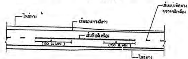
การตีเส้นจราจร กรณีความกว้างของช่องจราจรลดลง ไม่แสดงทางสวน
