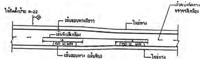
การตีเส้นจราจร กรณีความกว้างของช่องจราจรลดลง ไม่แสดงทางสวน
