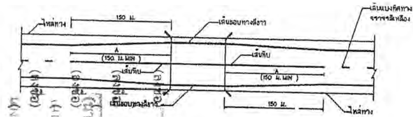
การตีเส้นจราจรกรณีความกว้างสะพานมากกว่าความกว้างผิวจราจรถนน ไม่แสดงทางสวน
