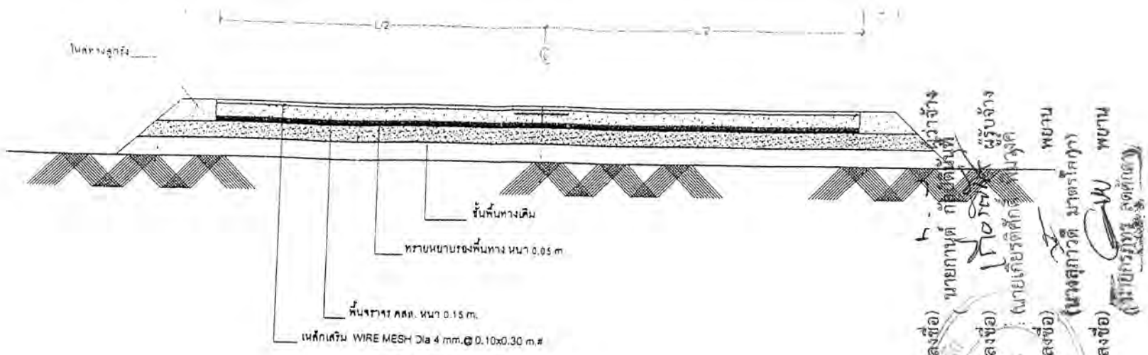
รูปตัดถนนคอนกรีตเสริมเหล็ก SCALE NO.
