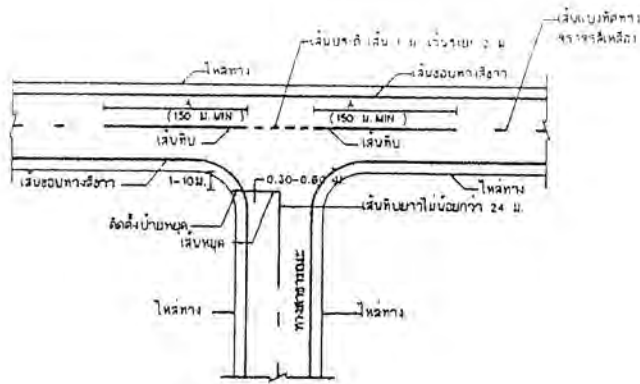
การตีเส้นจราจรทางแยก (ทางค้ำวางนึ่ง)
