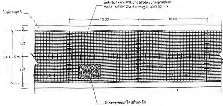
รูปแปลนแสดงการเสริมเหล็กและรอยต่อ SCALE NO.
