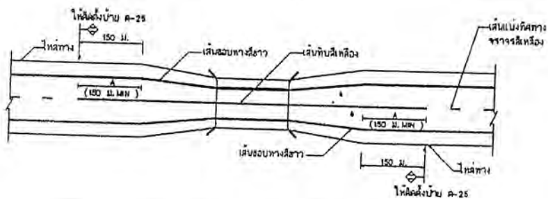
การตีเส้นจราจรกรณีความกว้างสะพานน้อยกว่าความกว้างผิวจราจรถนน ไม่แสดงขนาดส่วน
