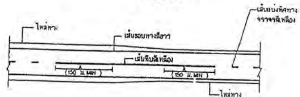
การตีเส้นจราจร กรณีความกว้างของช่องจราจรลดลง ไม่แสดงขนาดส่วน
