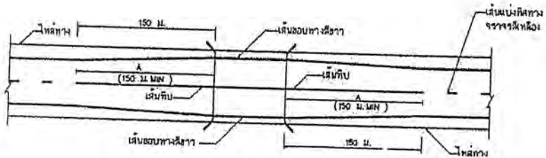
การตีเส้นจราจรกรณีความกว้างสะพานมากกว่าความกว้างผิวจราจรถนน ไม่แสดงขนาดส่วน
