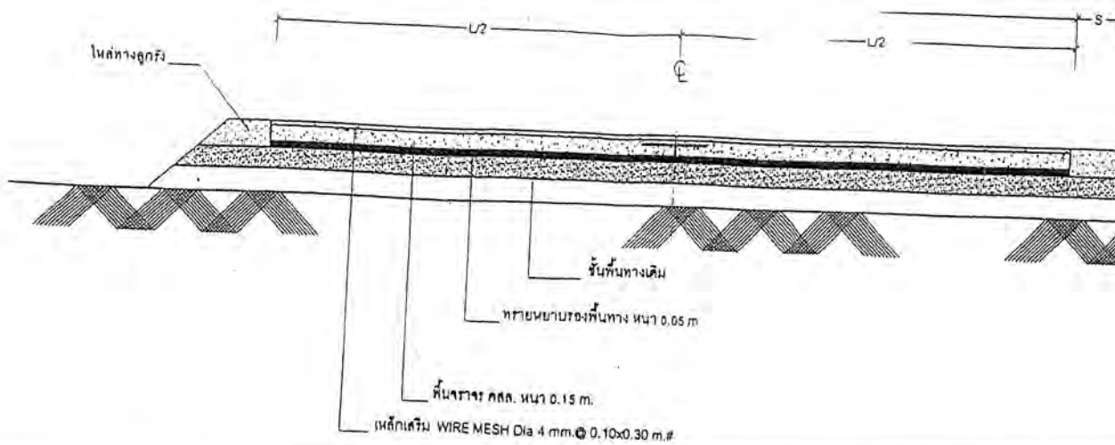
รูปตัดถนนคอนกรีตเสริมเหล็ก SCALE NO.
