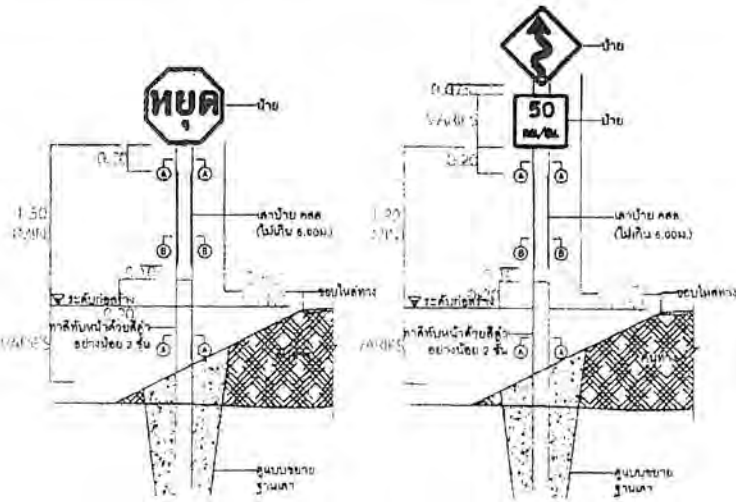
แสดงการติดตั้งป้ายและนำ ป้ายไม้กับป้ายเตือน
