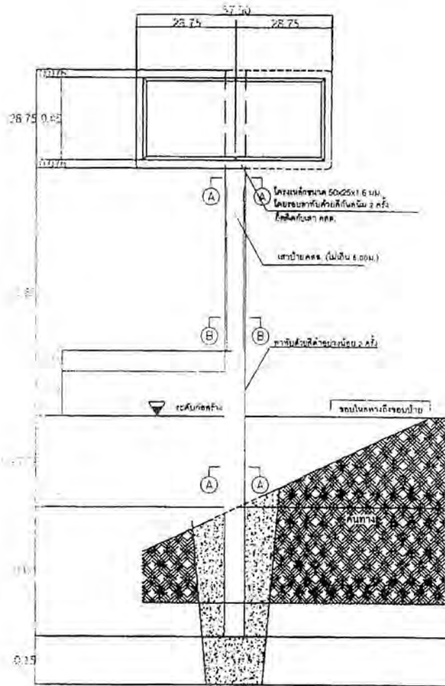
แบบแสดงการติดตั้งป้าย NOT TO SCALE
