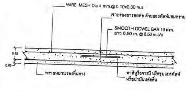
DETAIL 1. CONSTRUCTION JOINT (รอยต่อเพื่อการก่อสร้าง) SCALE NO.
