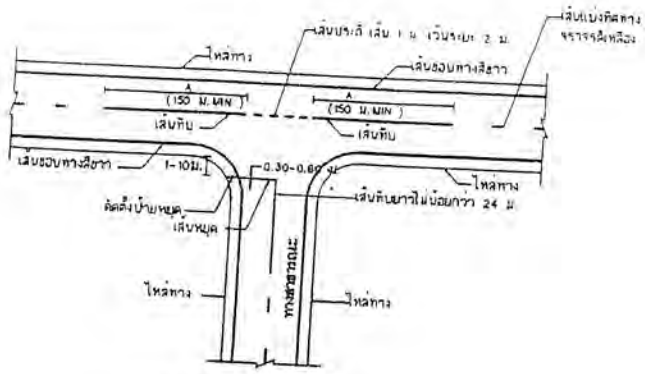
การตีเส้นจราจรทางแยก (ทางสายตรง)
