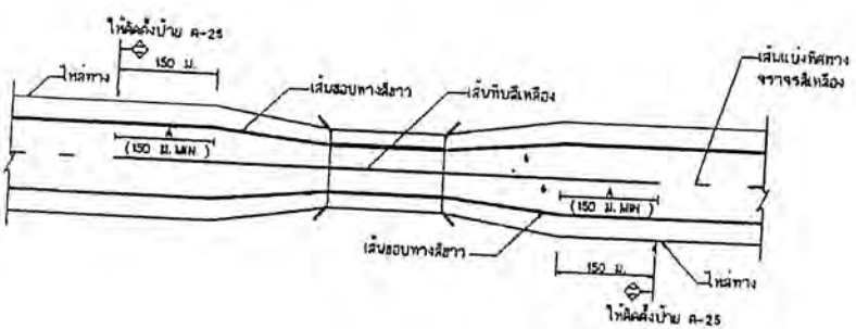
การตีเส้นจราจรกรณีความกว้างสะพานน้อยกว่าความกว้างผิวจราจรบน ไม่แสดงครุฑตัว
