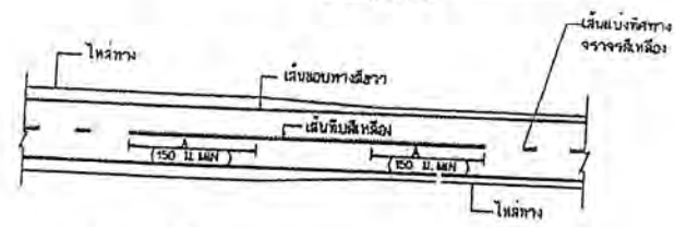
การตีเส้นจราจร กรณีความกว้างของไหล่ทางลดลง ไม่แสดงครุฑตัว
