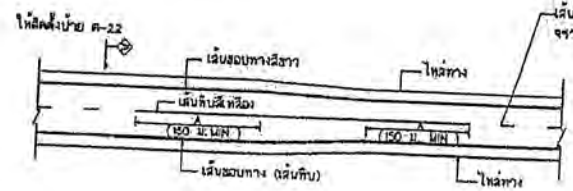
การตีเส้นจราจร กรณีความกว้างของช่องจราจรลดลง ไม่แสดงครุฑตัว
