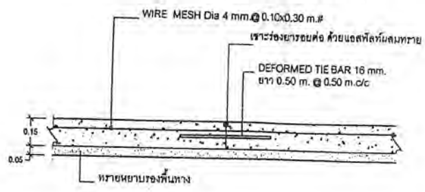
DETAIL 3. EXPANSION JOINT (รอยต่อเพื่อการขยายตัว) SCALE NO.
