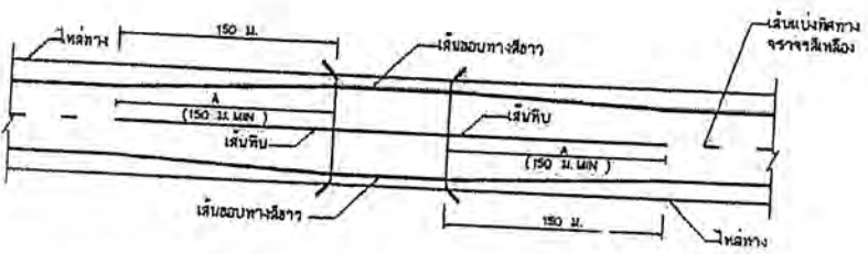
การตีเส้นจราจรกรณีความกว้างสะพานมากกว่าความกว้างผิวจราจรบน ไม่แสดงครุฑตัว
