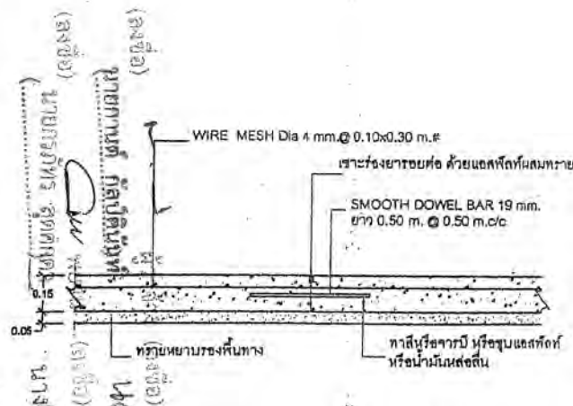
DETAIL. CONSTRUCTION JOINT (รอยต่อเพื่อการก่อสร้าง) SCALE NO.
