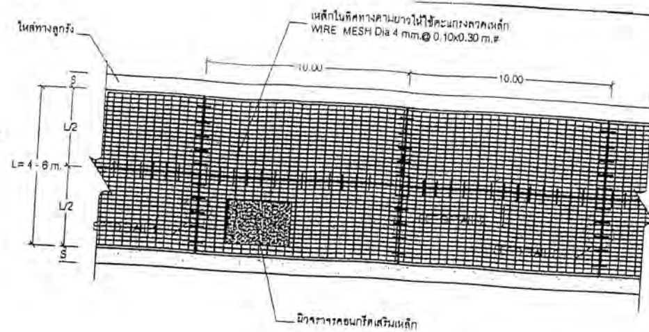
รูปแบบแสดงการเสริมเหล็กและรอยต่อ SCALE NO.
