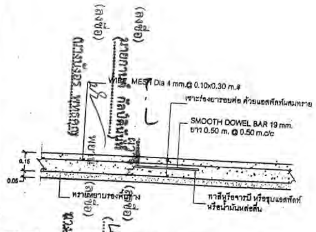
DETAIL. CONSTRUCTION JOINT (รอยต่อเพื่อการก่อสร้าง) SCALE NO.
