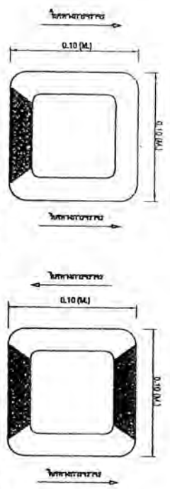
แปลนหน้าตัดของเสาเข็มคอนกรีตอัดแรง
