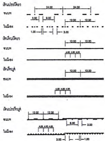
การติดตั้งปริมัณฑ์ที่เส้นศูนย์กลางทาง
