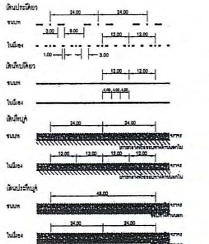
การติดตั้งปริมัณฑ์ที่เส้นแบ่งช่องจราจรและขอบทาง
