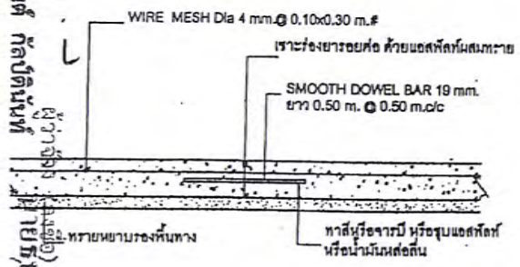
CONSTRUCTION JOINT (รอยต่อเพื่อการก่อสร้าง) SCALE NO.
