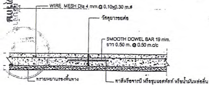
DETAIL 3. EXPANSION JOINT (รอยต่อเพื่อการขยายตัว) SCALE NO.
