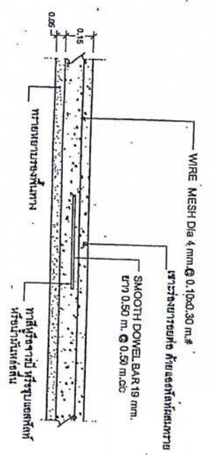
DETAIL. 2. LONGITUDINAL JOINT (รอยต่อยาว) SCALE NO.
