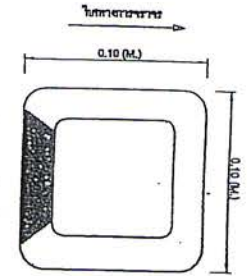
แบบแปลนค้ำยันชั่วคราวแบบรับน้ำหนักด้านเดียว
