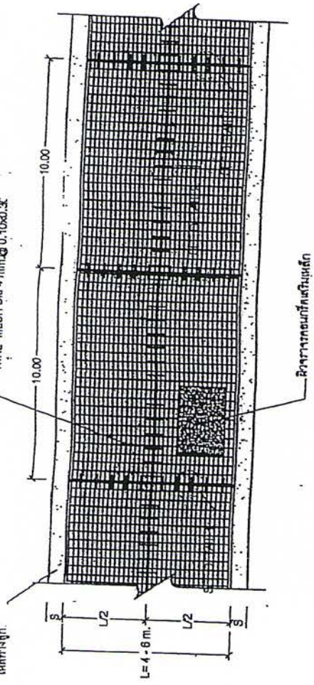
รูปแบบแผนแสดงการเสริมเหล็กและรอยต่อ SCALE NO.
