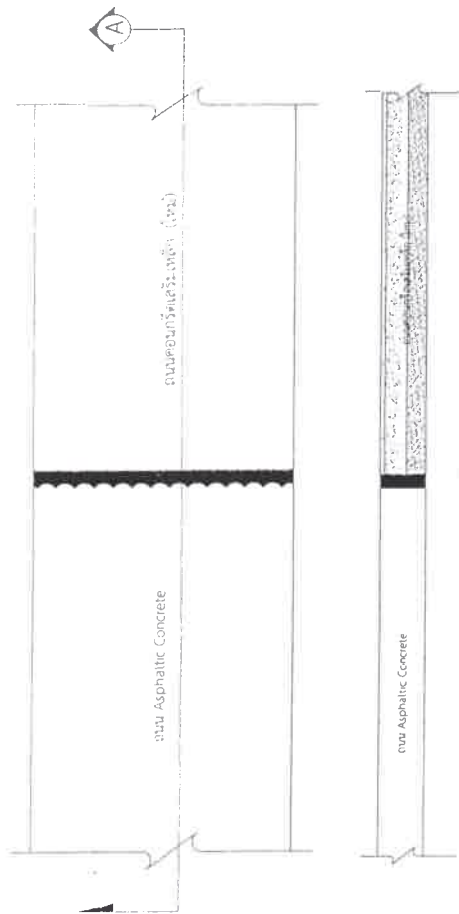
รูปตัด (A) SCALE NO. _____ กรณีเชื่อมกับถนน Asphaltic Concrete ให้เว้นระยะห่างไม่น้อยกว่า 1C ซม แล้วเชื่อมรอยต่อด้วย ยางมะตอย หรือ พรีมิกซ์
