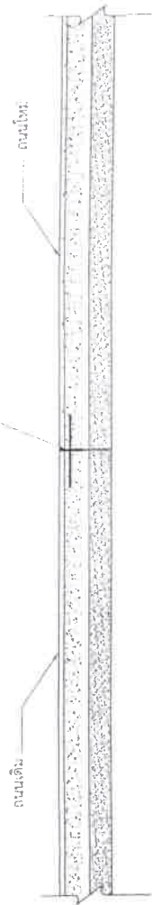
แบบรอยต่อถนนเดิม / ถนนใหม่ SCALE NO. _____ กรณีเชื่อมกับถนน คอนกรีตเสริมเหล็ก (เดิม)
