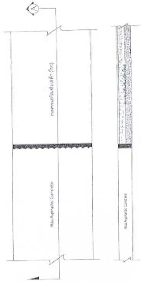
รูปตัด A
