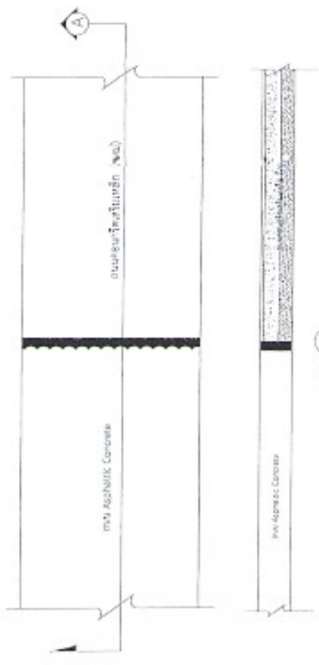
รูปตัด A-A SCALE NO. _____
