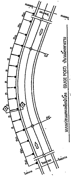
การติดตั้ง หลุมเจาะเข็ม (GUIDE POST) บริเวณทางรถไฟ (ใช้สำหรับติดตั้งสายเคเบิลสายเคเบิล)
