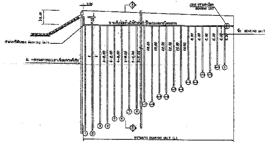
รูปตัด ๑ - ๑ แสดงตำแหน่งเสาเข็ม
