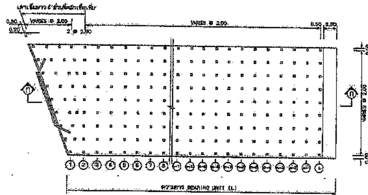
แบบแสดงตำแหน่งเสาเข็ม (กรณีสะพานเอียงกับลำน้ำ)
