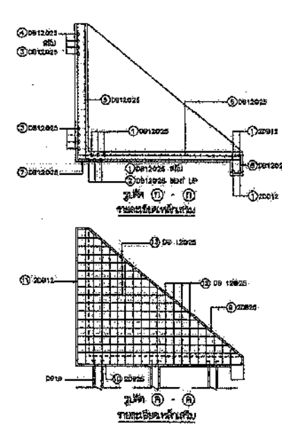
รูปตัด (ก) - (ข) รายละเอียดโครงสร้าง
