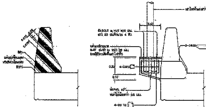
ส่วนหน้าของสะพาน ภาพร่างแบบที่ 2
