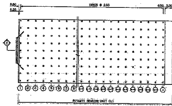
แบบแสดงตำแหน่งเสาเข็ม (กรณีสะพานตั้งฉากกับลำน้ำ)
