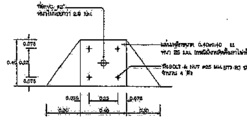
ส่วนหน้าของสะพาน ภาพร่างแบบที่ 1
