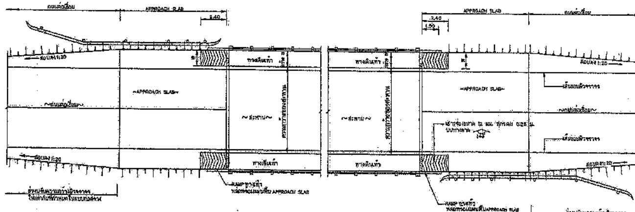
แบบรูปทิว URB APPROACH SLAB
