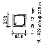
แบบแปลน ฐานราก F1 Scale 1:25
