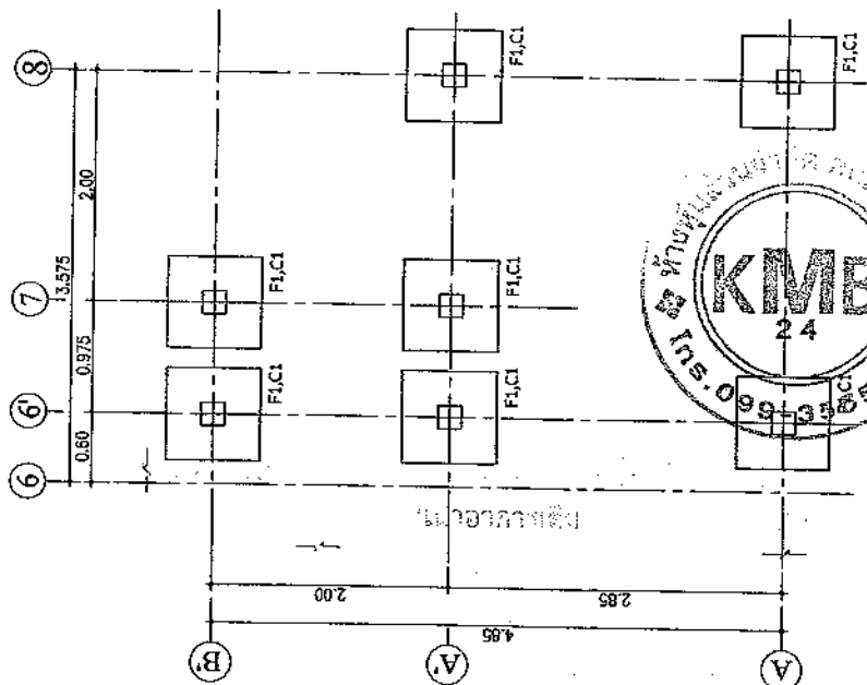
แบบแปลนฐานราก F1 Scale 1:25
