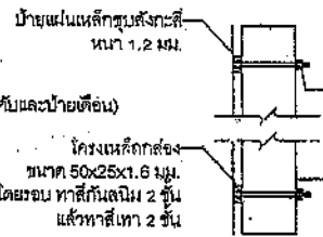
แสดงการติดตั้งโครงเหล็กกล่องกับเสาป้าย
