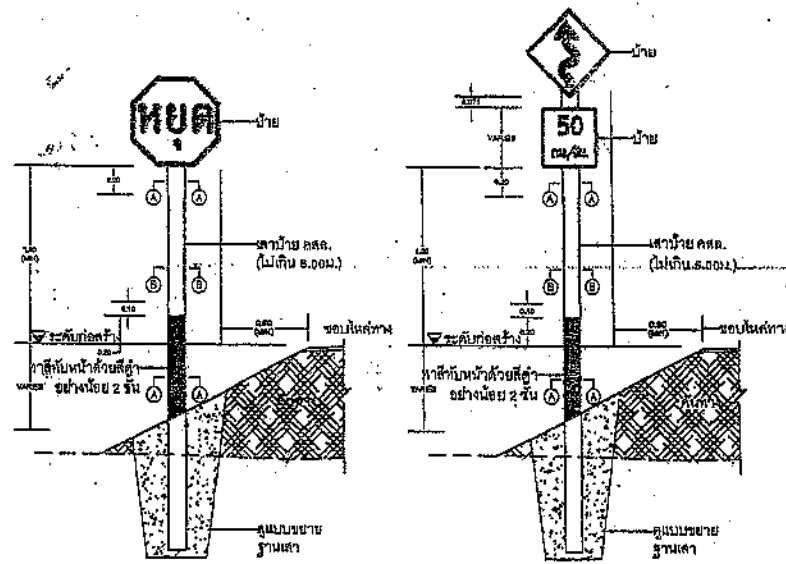
แสดงการติดตั้งป้ายและนำป้ายไม้ค้ำและป้ายเตือน
