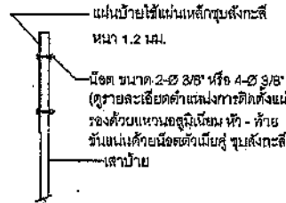
แสดงการติดตั้งป้ายไม้ค้ำ ป้ายเตือน
