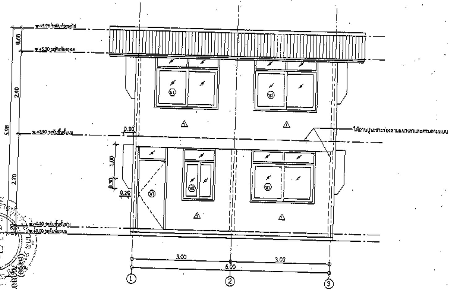
รูปด้าน 1 มาตรฐาน 1: 50
