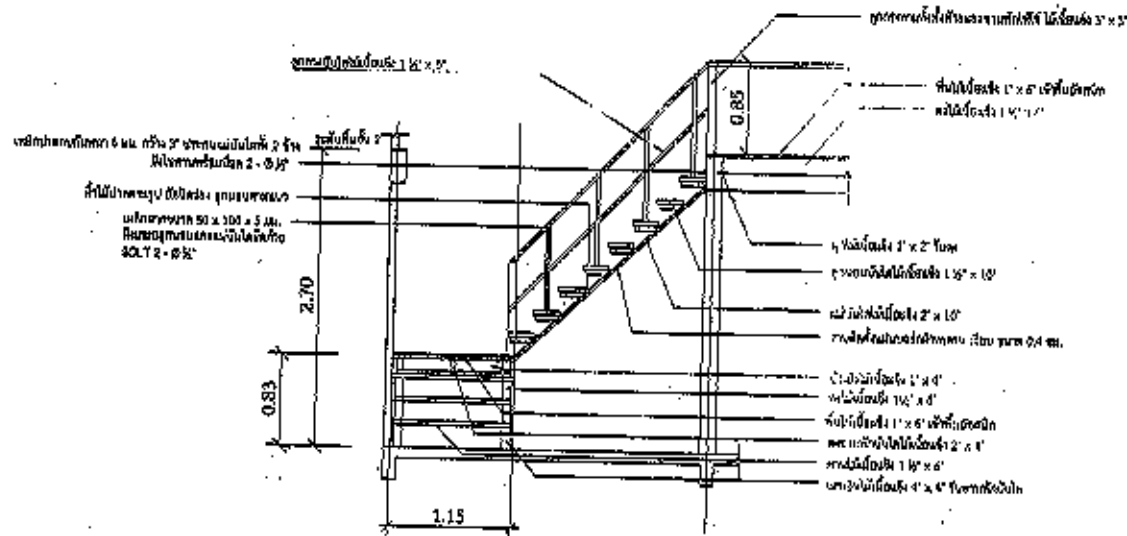
มาตรา ๗๖ 1:50
