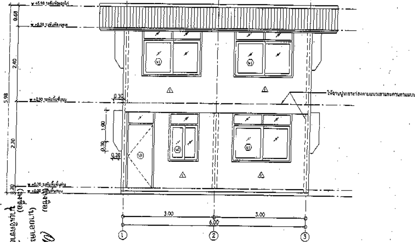
รูปด้าน 2
