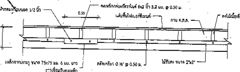
รูปตัด A มาตราส่วน NOT TO SCALE
