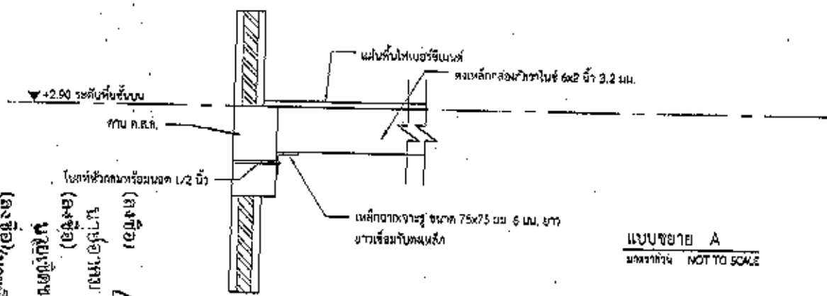
แบบขยายขยายพื้น มาตราส่วน NOT TO SCALE
