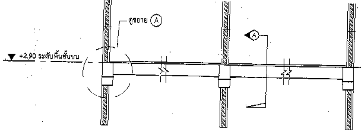
แบบขยายขยายพื้น มาตราส่วน NOT TO SCALE
