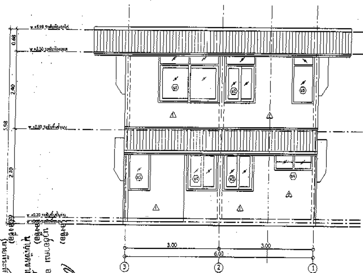
รูปด้าน ๓ มาตราส่วน 1 : 50
